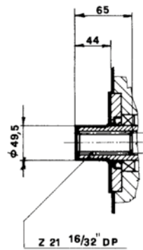
90004 Hembra Larga Z-21T
